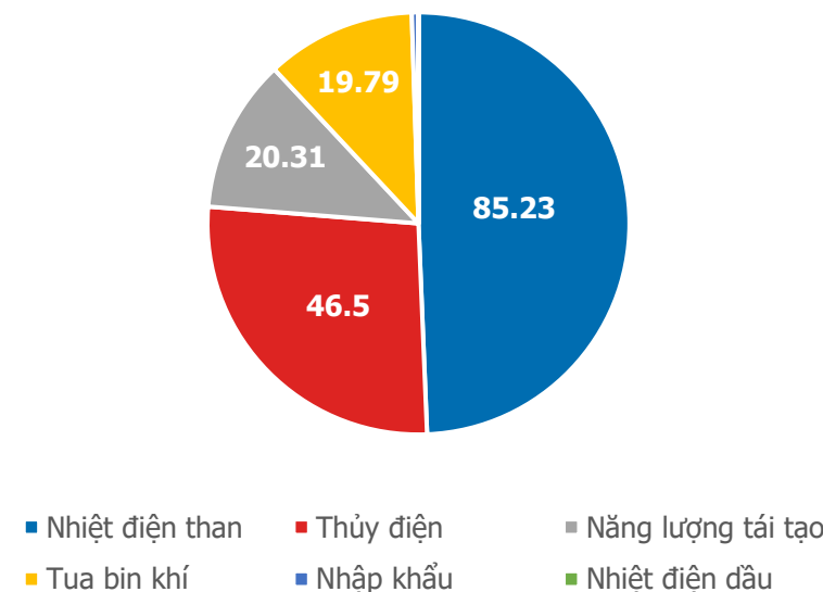
Sản lượng điện sản xuất lũy kế 8 tháng 2021 (Tỷ kWh)
